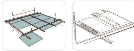
CLIP-IN Tavan Uygulama
