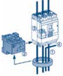
⊙ Toroid ⊙ Vigirex röle ⊙ MX bobini ⊙ Nötr
